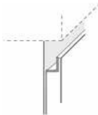
GOLA PIATTA Art. 485
