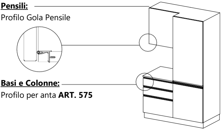
Profilo ART. 575 Orizzontale
